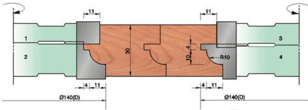
TF607B D140*d30*Z4 1SET/4PCS
