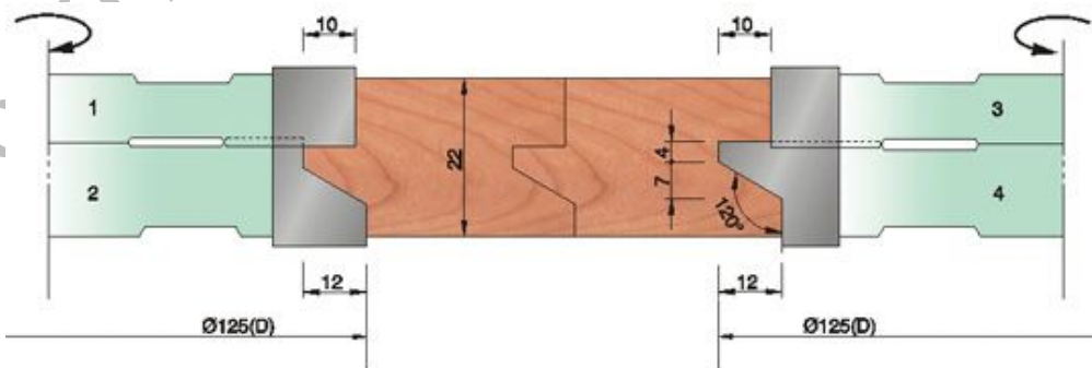
TF606F D125*d35*Z4 1SET/4PCS
