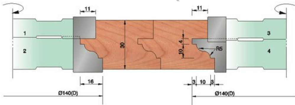
TF607C D140*d30*Z4 1SET/4PCS
