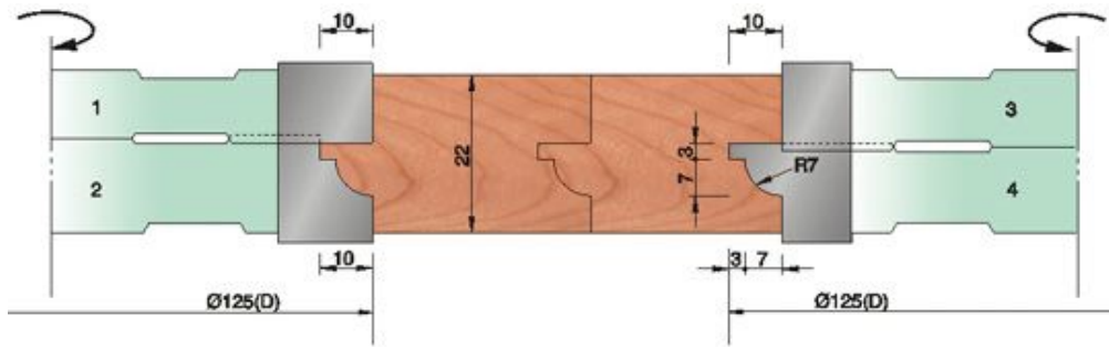
TF607A D140*d30*Z4 1SET/4PCS
