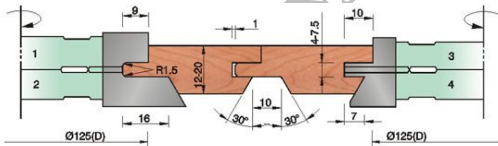
TF601PD125*d40*Z4/Z6 1SET/4PCS
